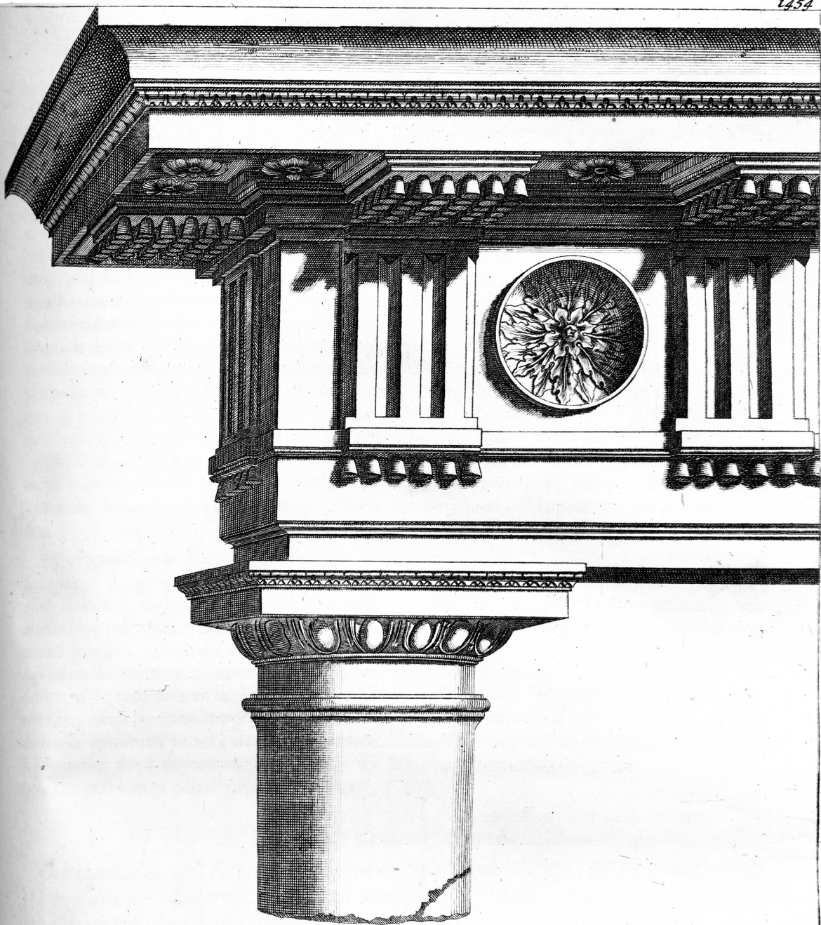
Aal-oud voorbeeld der Dorische Bouw-orden door Pijrrus Ligorius gemeen-gemaakt.
